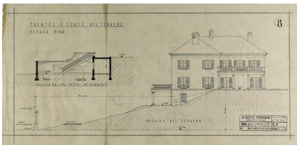
Plano de Frentes y Corte del terreno, Arq. Alberto Prebisch.
